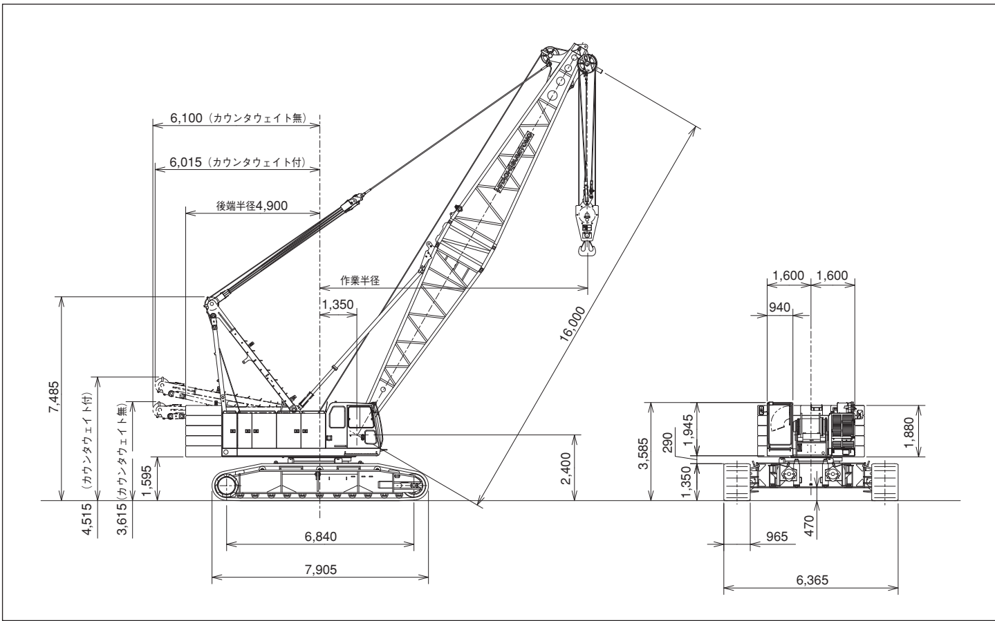
■寸法図
